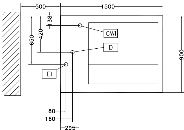
Boven aanzicht
